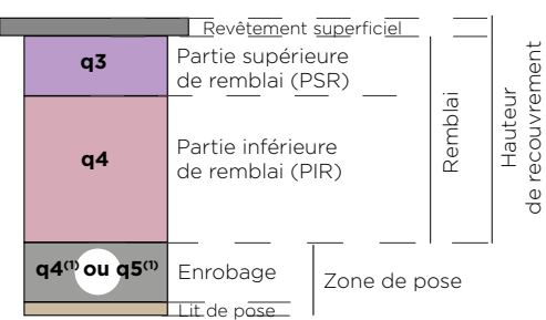
COUPE TROTTOIR
