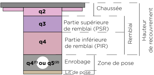
COUPE CHAUSSEE
